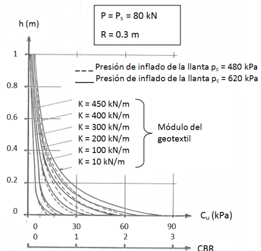
Figura 7. Gráficos método de Giroud y Noiray. Fuente: [5]
