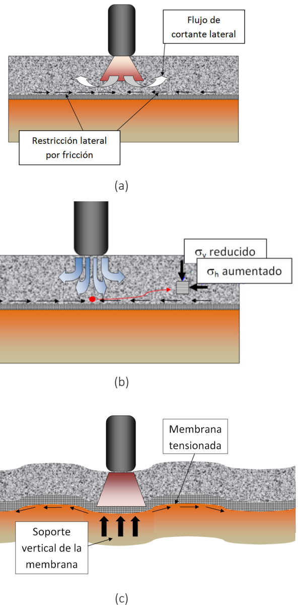
Figura 1. Mecanismos de refuerzo de geosintéticos en pavimentos (a) Restricción lateral, (b) Incremento en la capacidad de soporte y (c) Efecto de membrana.
