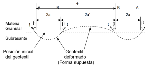
Figura 4. Geometría de deformación del Geotextil. Fuente: [5]
