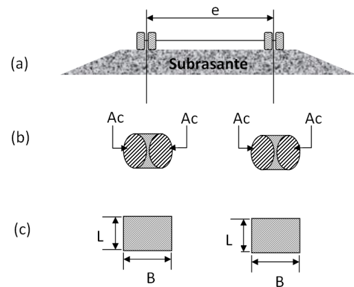
Figura 2. Geometría del eje del vehículo y definición del área de contacto: (a) Geometría del eje vehicular; (b) Áreas de contacto; (c) Área de contacto equivalente. Fuente: [5, modificada y adaptada por autor]
