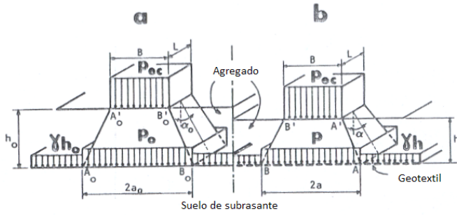
Figura 3. Distribución de la carga en la capa de agregado: (a) caso sin geosintético, (b) caso con geosintético Fuente: [5]
